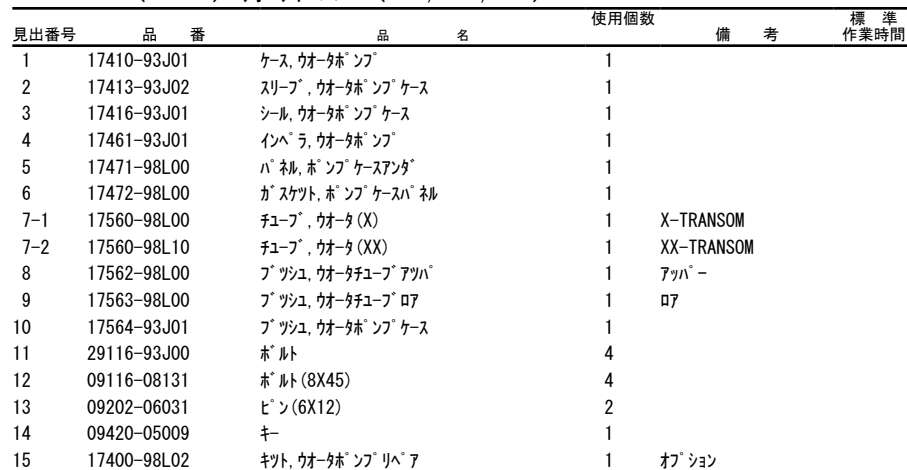
FIG. 160A (1-C-6) ウォータホップ (020, 021, 022)
