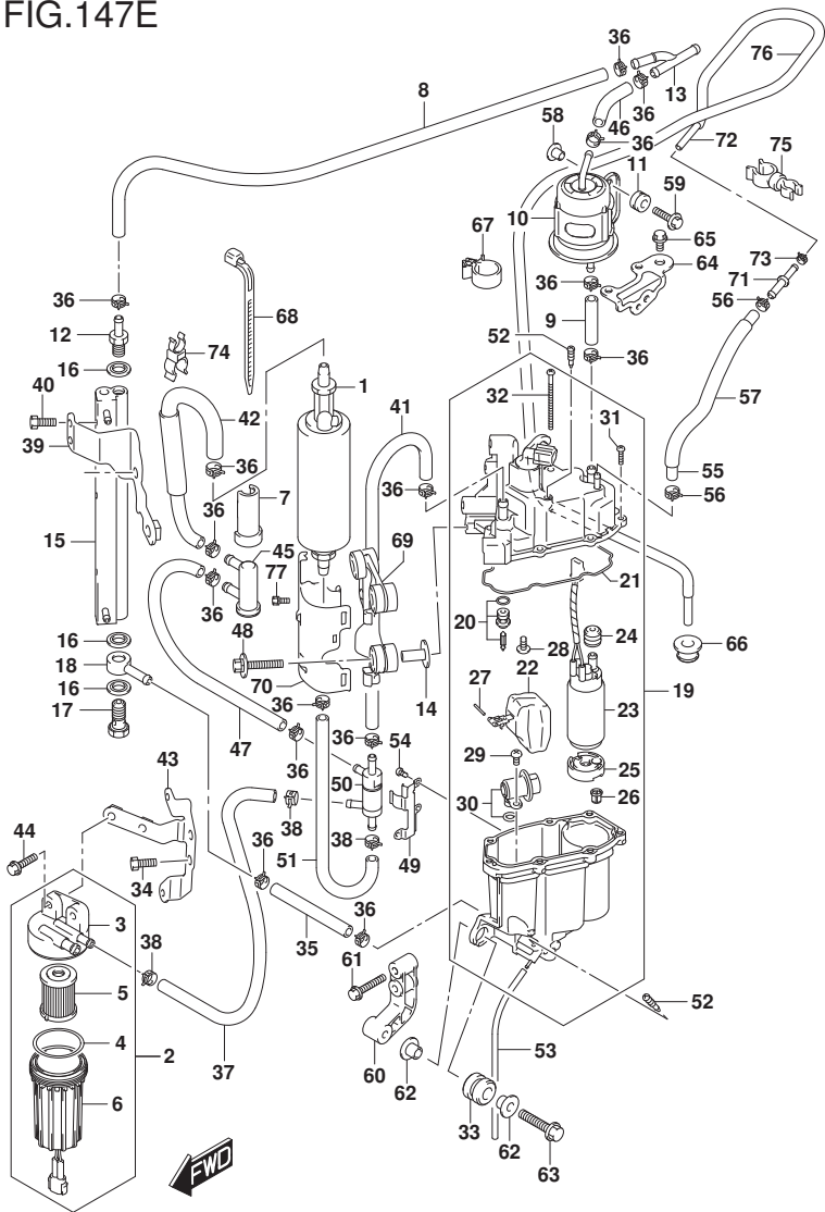
FIG. 147E (1-E-6) フューエルポンプ / フューエルベ-ハセパレータ (SEE NOTE 1)
