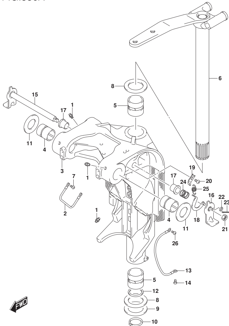
FIG. 336A (1-I-11) スイベルブ ラケット (L-TRANSOM:DF200T)
