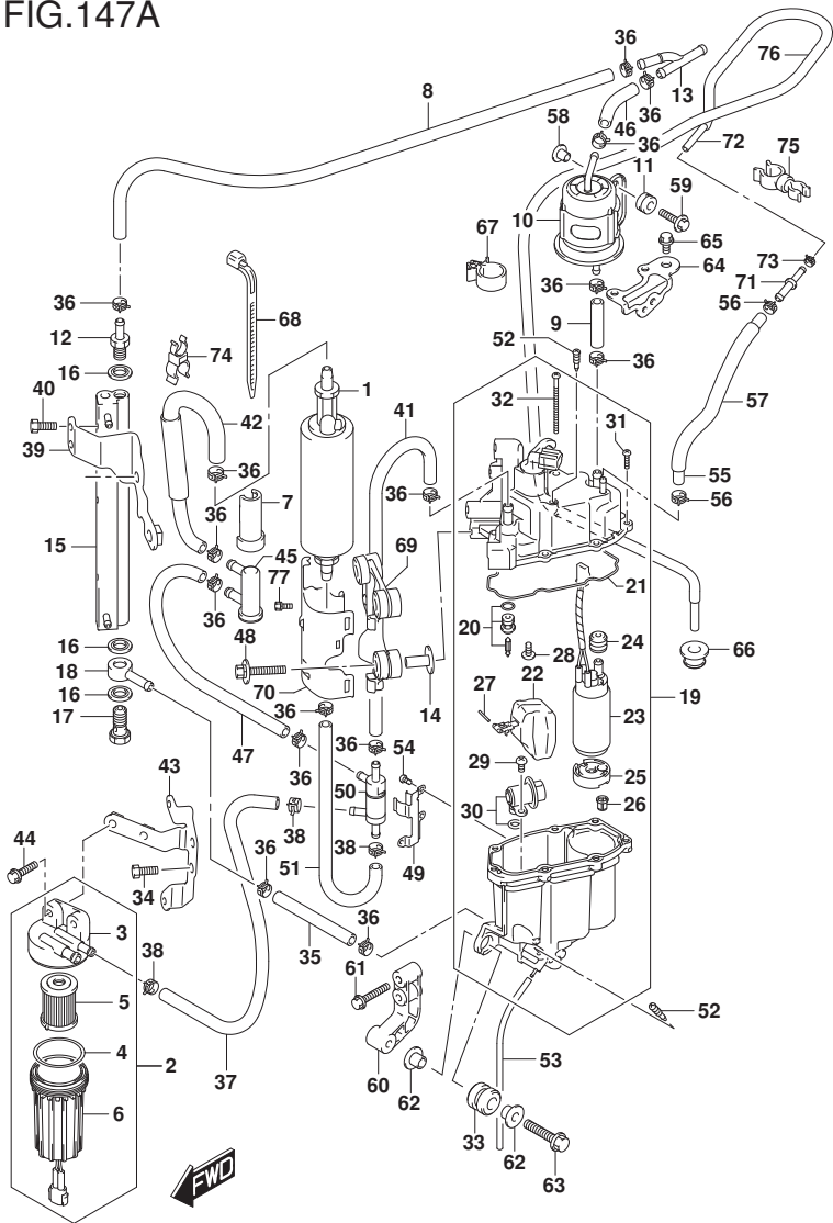
FIG. 147A (1-D-8) フューエルポンプ / フューエルベ-ハセパレータ (SEE NOTE 1)
