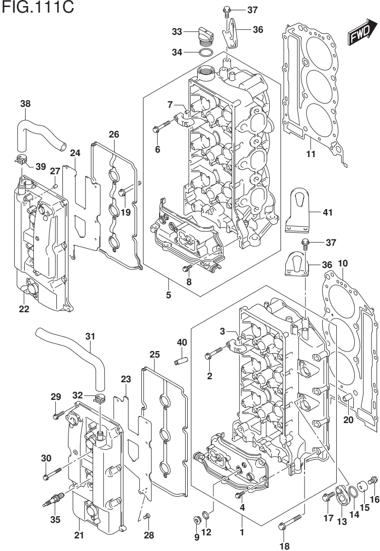
FIG. 111C (1-B-7) シリンダーヘッド (DF275ST)
