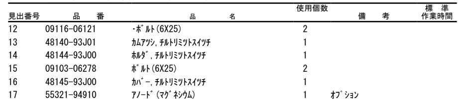
FIG. 335A (1-I-7) クランプ フ ラケット (L-TRANSOM:DF200T)
