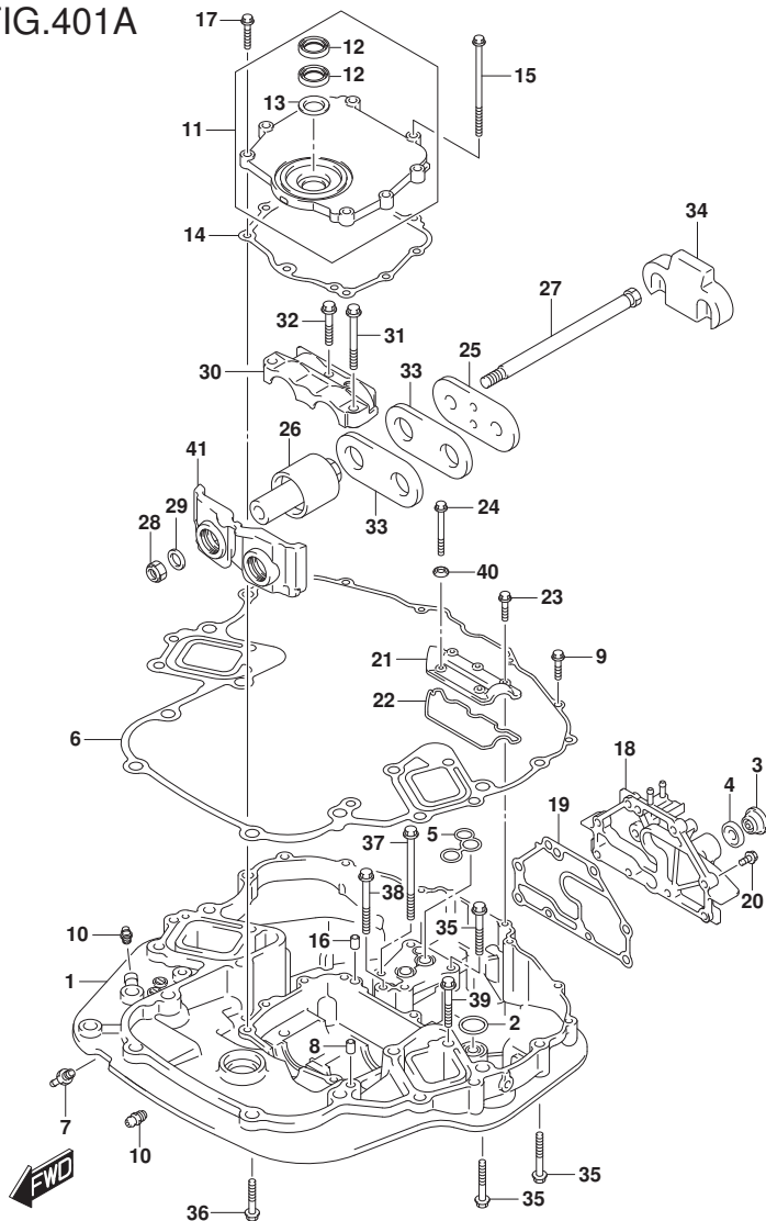
FIG. 401A (1-K-10) エンジンホルダー (DF200T)
