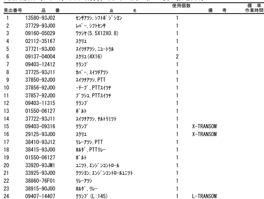
FIG. 326A (1-F-7) PTT スイッチ/エンジン コントロール ユニット (DF200T)
