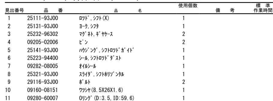
FIG. 206A (1-E-3) クラッチロッド * (DF200T)
