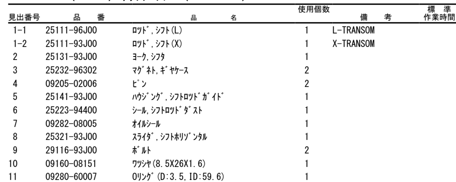
FIG. 206B (1-D-2) クラッチロッド * (DF200AST)
